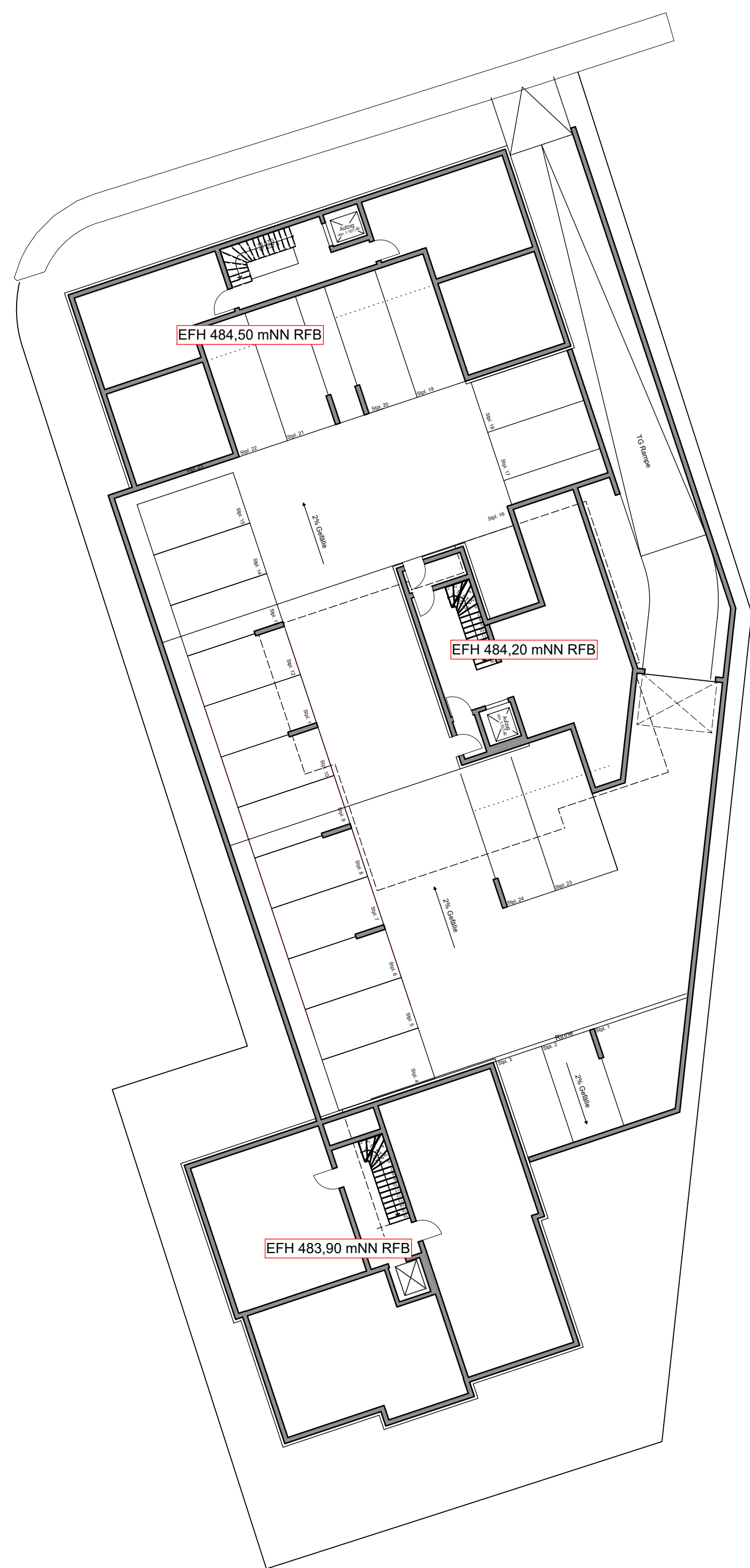
Tiefgarage M 1:200
