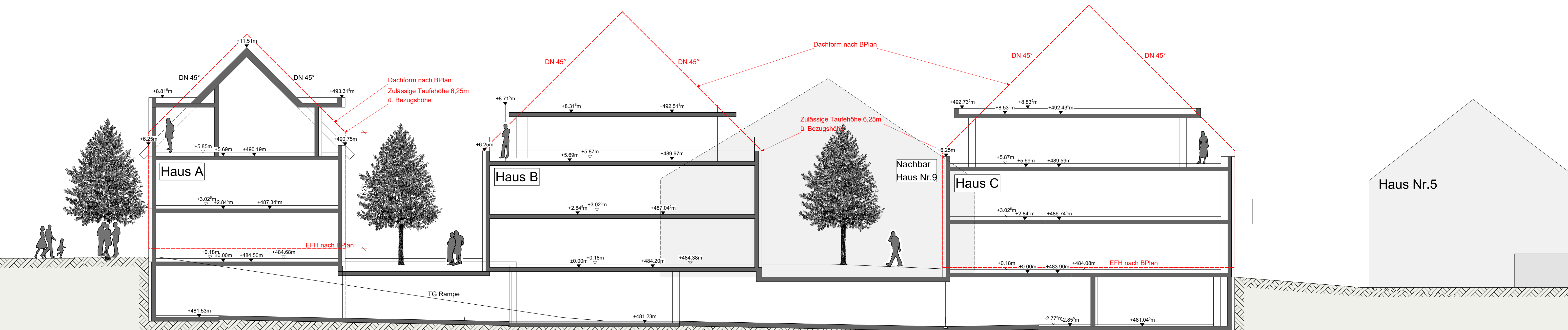
Schnitt A-A
