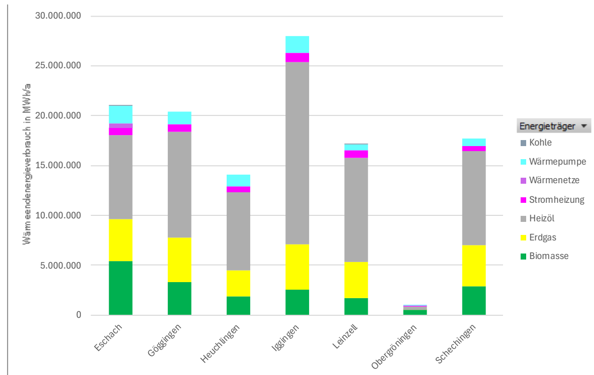
Abbildung 15 Wärmeeindenergieverbrauch nach Energieträgern
