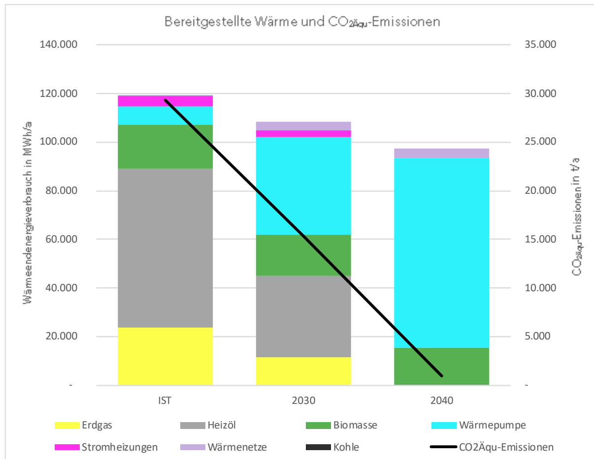
Abbildung 28 Entwicklung des Wärmeendenergiebedarfs und Emissionen nach Heiztechnologien in MWh & der CO 2 Äqu-Emissionen in t (Gesamtkonvoi)
