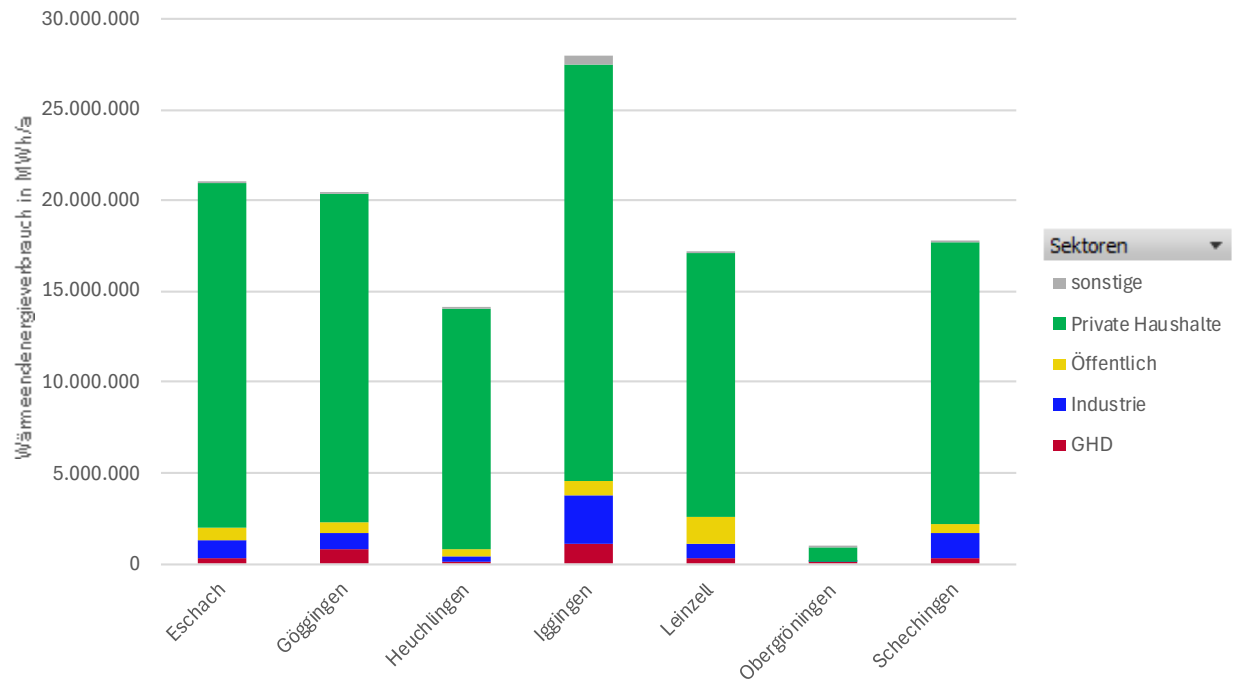
Abbildung 16 Wärmeendenergieverbrauch nach Sektoren
