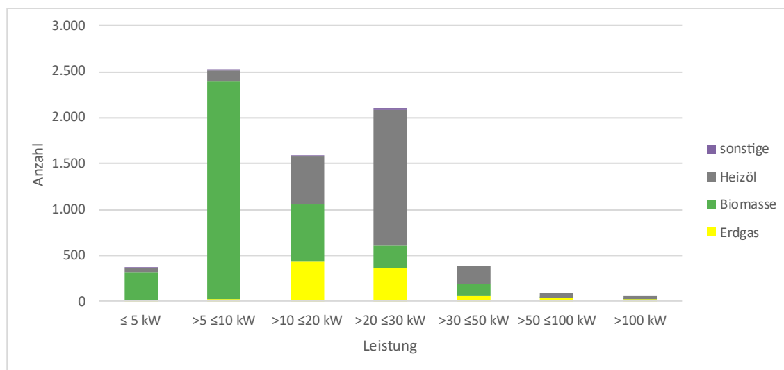
Abbildung 13 Leistung der Feuerungsanlagen nach Brennstoffen und Leistungsklassen
