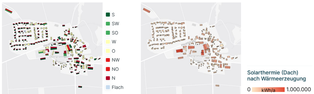
Abbildung 21 Solarthermiepotezial auf Dächern (Obergröningen) (links: Dachausrichtung; rechts: Wärmeerzeugung p.a.) (eigene Darstellung, Datenquelle: LGL, www.lgl-bw.de , dl-de/by-2-0")
