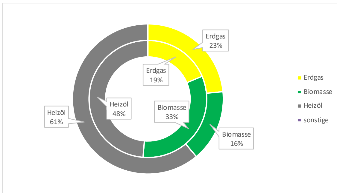
Abbildung 11 Summe der Leistungen aller Feuerungsanlagen (innen) sowie der Zentralheizungen (außen) im Konvoi
