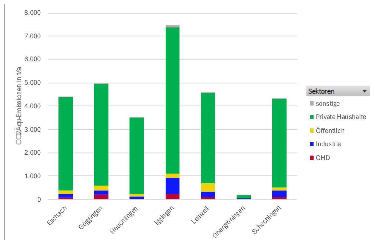
Abbildung 18 THG-Emissionen nach Sektoren
