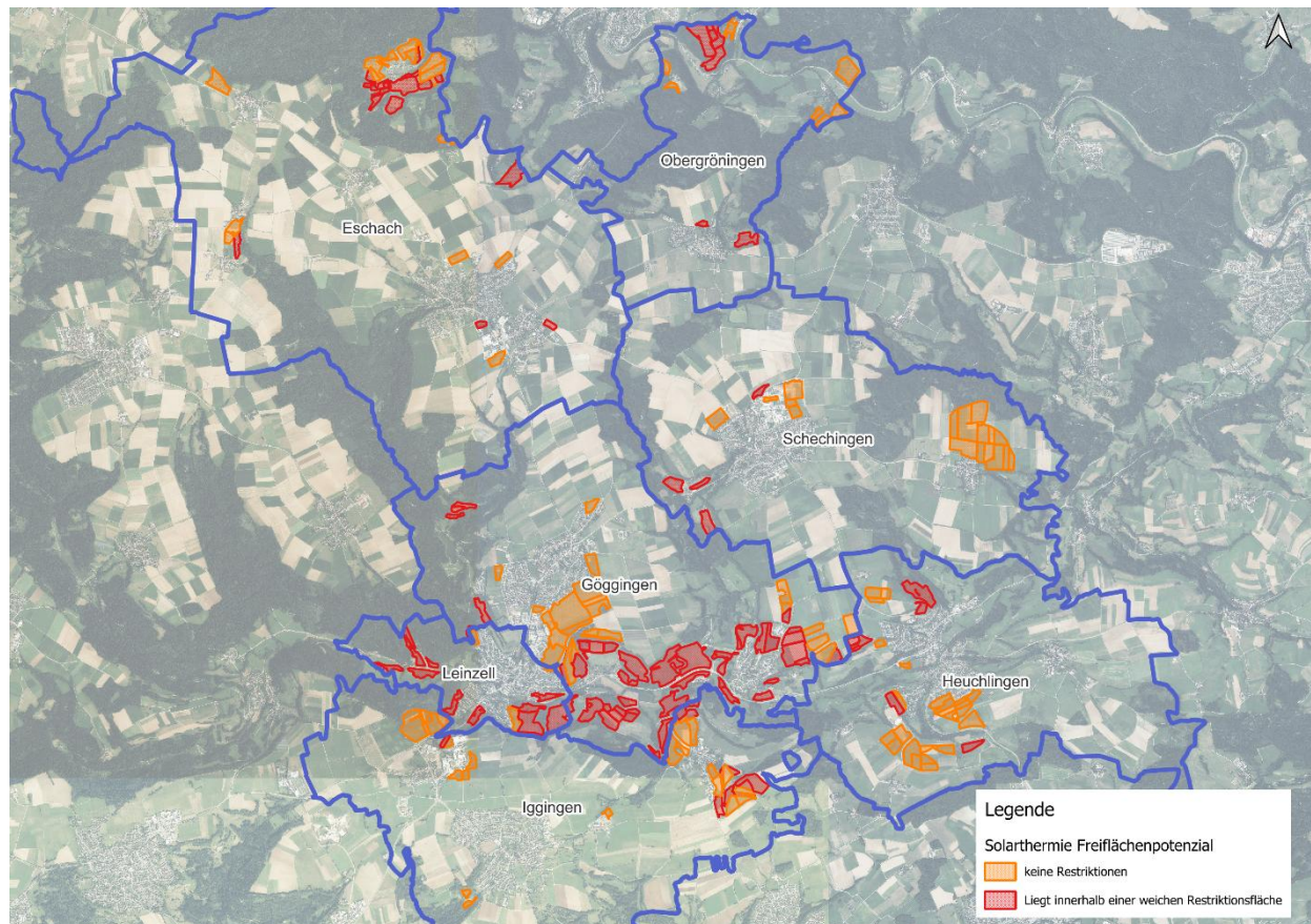
Abbildung 22 Solarthermiefreiflächenpotenzial auf Freiflächen (eigene Darstellung, Datenquelle: LGL, www.lgl-bw.de , dl-de/by-2.0*)
