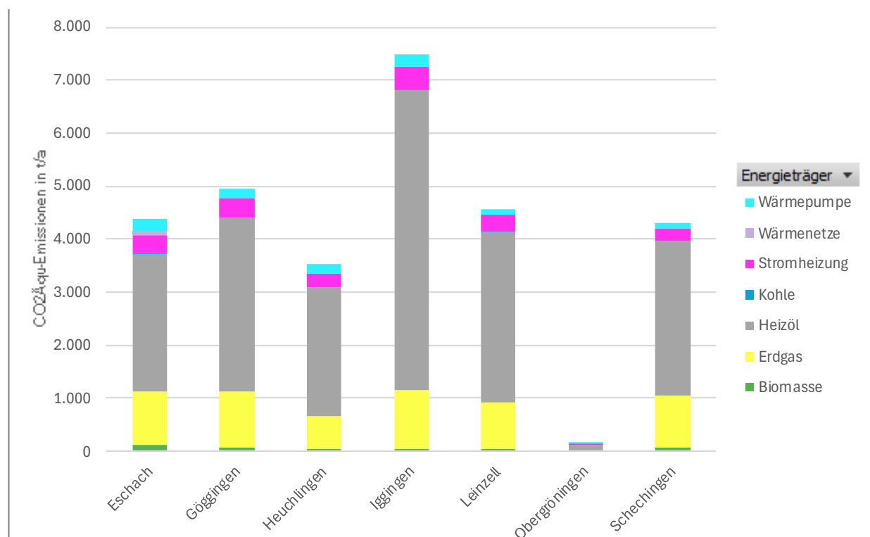
Abbildung 17 THG-Emissionen nach Energieträgern
