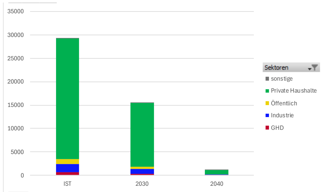
Abbildung 30 Entwicklung der THG-Emissionen nach Sektor in t CO 2 (Gesamtkonvoi)
