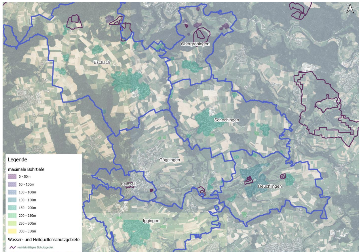
Abbildung 23 Flächenhafte Darstellung des möglicher Geothermie-Bohrtiefen & wasserschutzrechtlicher Restriktionen (eigene Darstellung, Datenquellen: LGL, www.lgl-bw.de , dl-de/by-2-0 und (KEA-BW, Universität Groningen, Hochschule Biberach, 2023))
