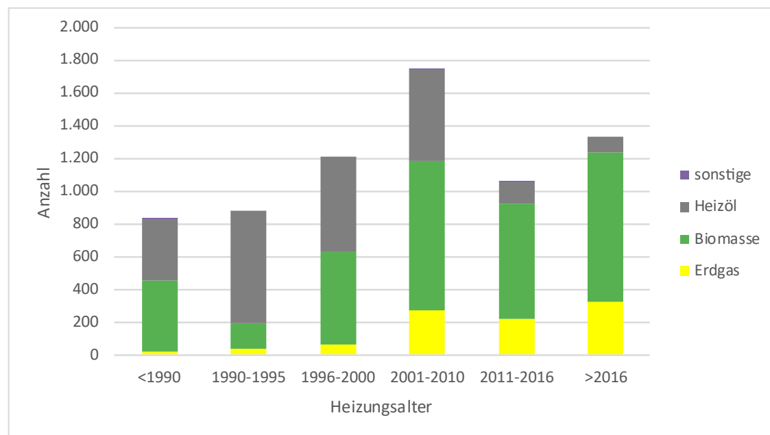
Abbildung 12 Altersverteilung aller Feuerungsanlagen nach Brennstoff
