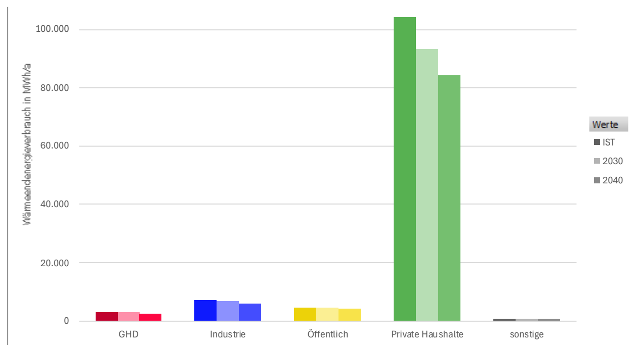
Abbildung 20 Energieeinsparungen nach Sektoren (2030 und 2040)
